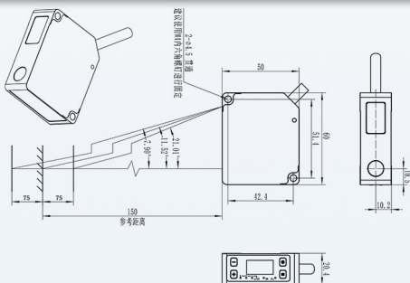
M3-150参数表
