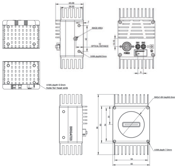
图2 LCP-M04K05CX-H300K-0507
